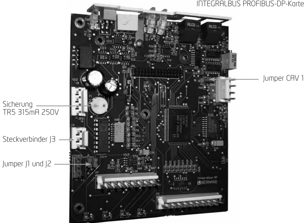
INTEGRALBUS PROFIBUS-DP-Karte
