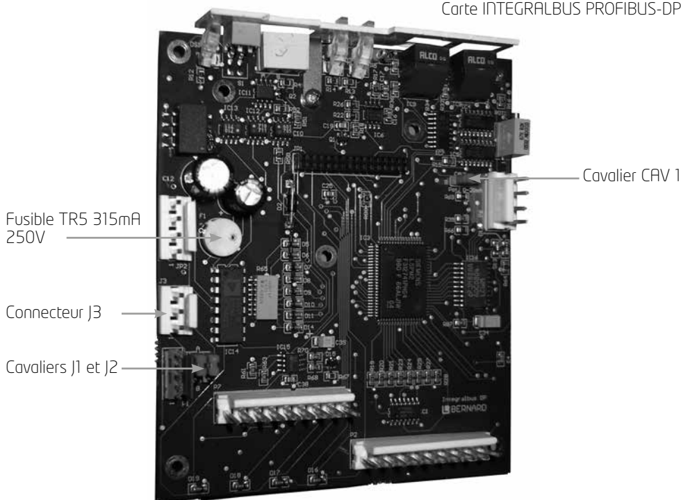
Carte INTEGRALBUS PROFIBUS-DP
